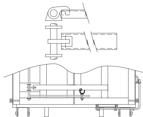
Barn door locking gear
